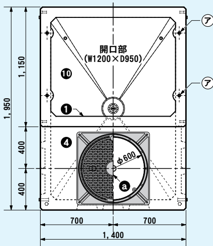
盤前面側
