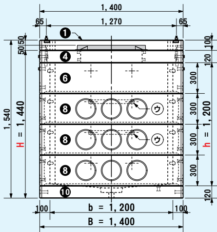
盤前面側
