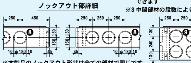
ロックアウト部詳細
