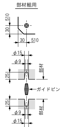
ガイドピン部詳細 ( 尺度 1 : 8 )
